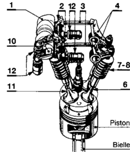
Mécanisme de commande de soupapes
